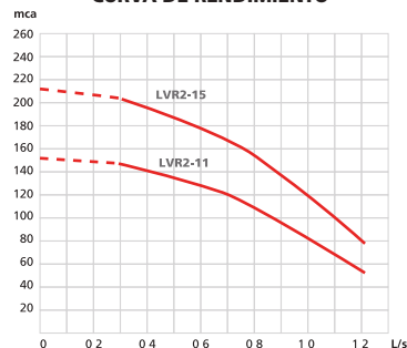
CURVA DE RENDIMIENTO
