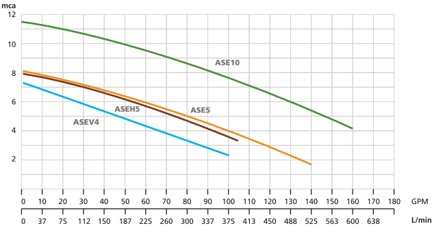
CURVA DE RENDIMIENTO
