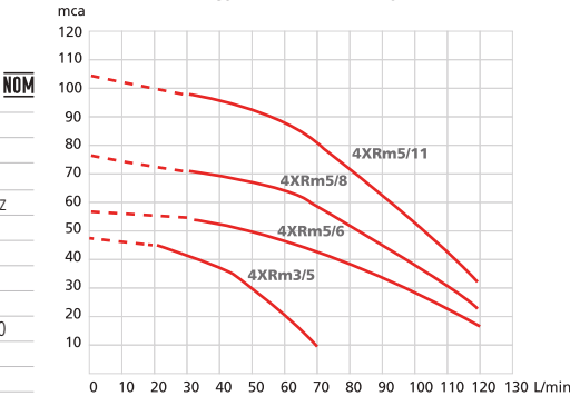
CURVA DE RENDIMIENTO
