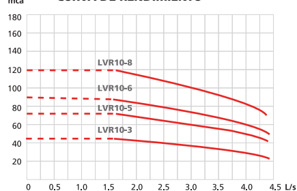
CURVA DE RENDIMIENTO
